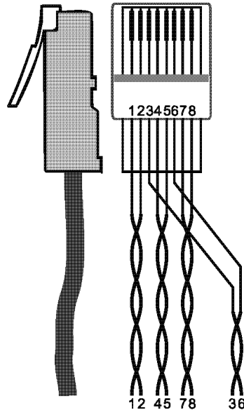
Рис. 3. Разводка кабеля на разъем RJ-45
