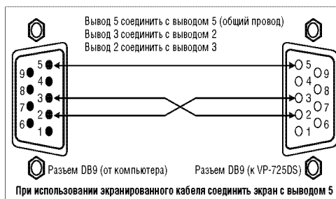
Рис. 2. Подключение к компьютеру
