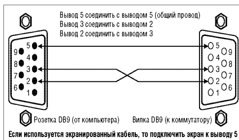
Рис. 10. Подключение к компьютеру
