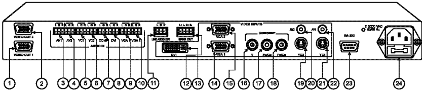
Рис. 8. Задняя панель VP-724xl
